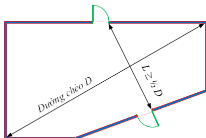
c) Xác định khoảng phân tán của các lối ra thoát nạn trong một số trường hợp mặt bằng phức tạp
